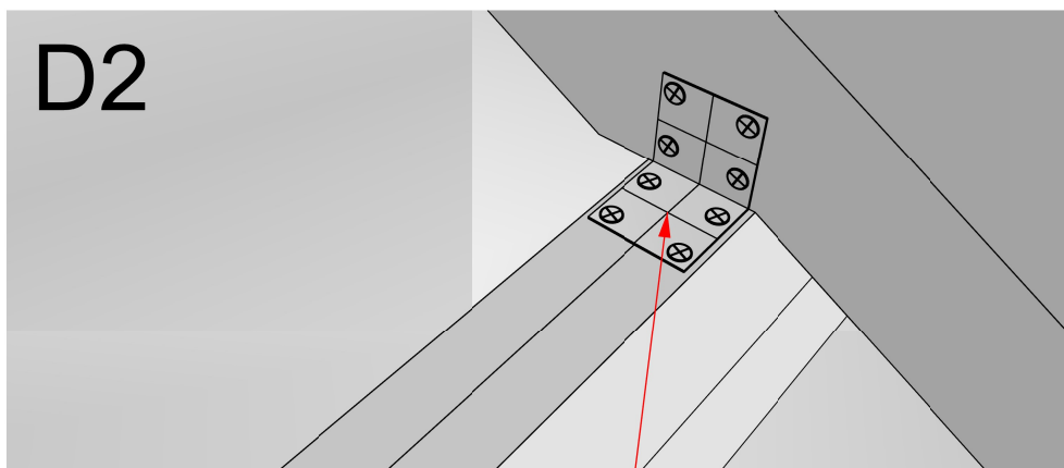
40x40 vinkel. 8 stk. 5x40mm. På begge sider af spær
