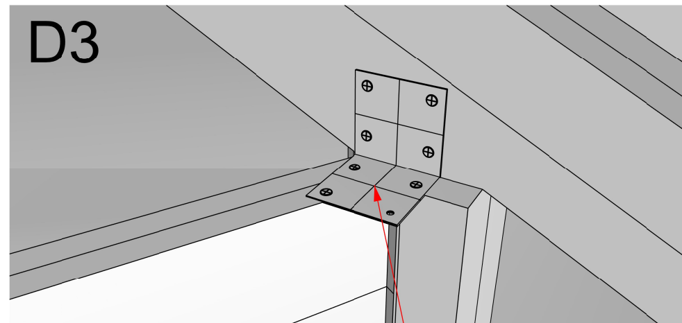
70x70 vinkel. 8 stk. 4x40mm. På begge sider af spær
